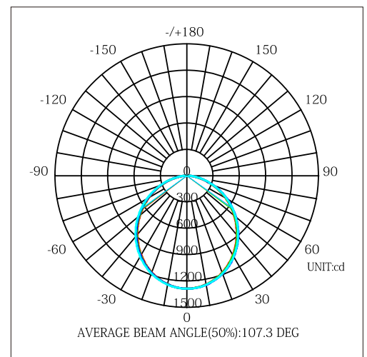
配光曲线及光强度分布图
