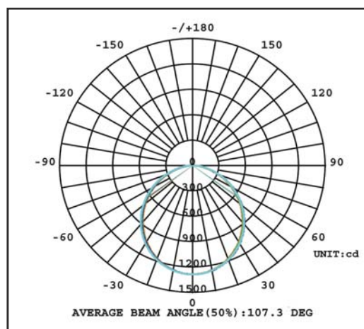
配光曲线和光强度分布图
