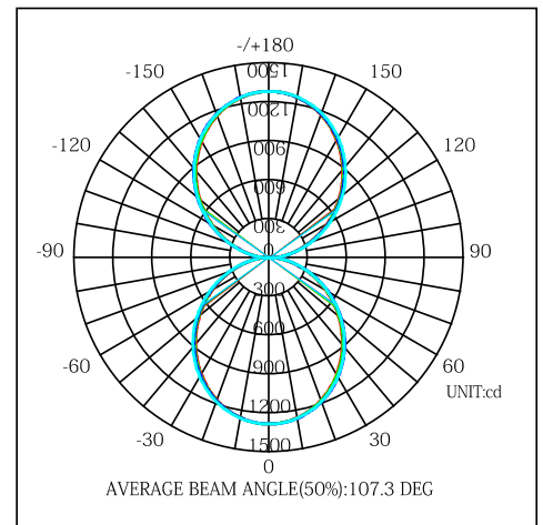
配光曲线及光强度分布图
